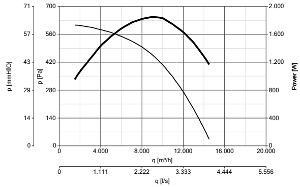
VORT QBK SAL-KC EVO 315 T2 1,5kW codice 43164
