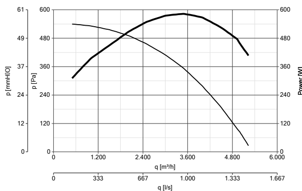
VORT QBK SAL-KC EVO 500 T4 1,5kW codice 43159
