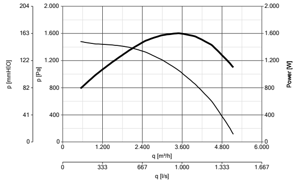
VORT QBK SAL-KC EVO 355 M4 0,25kW codice 43154
