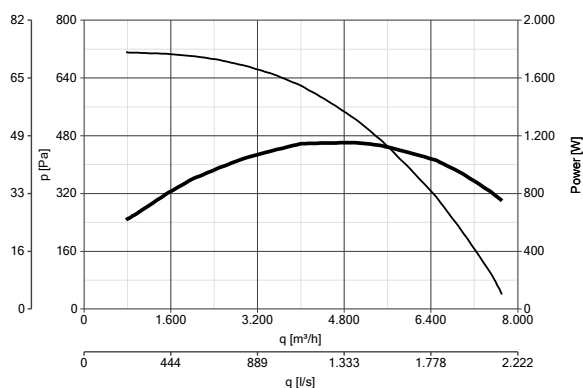
VORT QBK SAL-KC EVO 500 T6 0,55kW codice 43160
