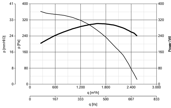
VORT QBK SAL-KC EVO 315 T4 0,25kW codice 43153
