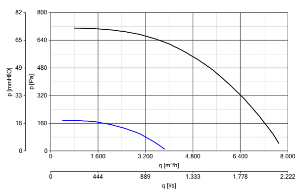
VORT QBK SAL-KC EVO 450 T4/8 1,1/0,18kW codice 43168
