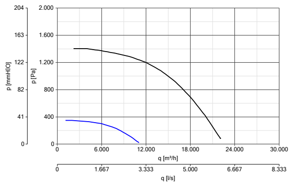
VORT QBK SAL-KC EVO 630 T4/8 5,5/1,1kW codice 43171
