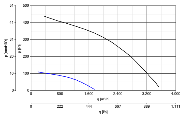
VORT QBK SAL-KC EVO 355 T4/8 0,25/0,03kW codice 43166
