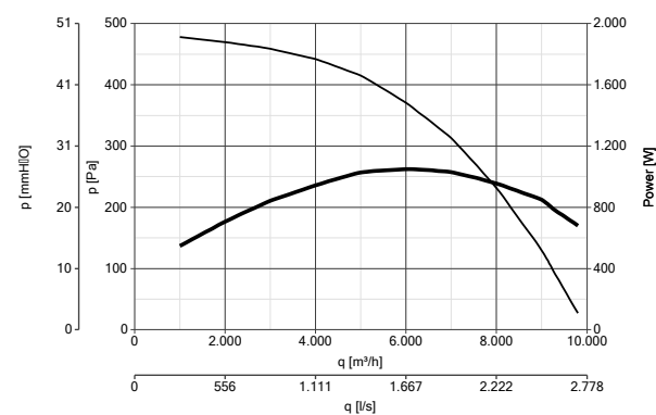
VORT QBK SAL-KC EVO 560 T6 1,1kW codice 43162
